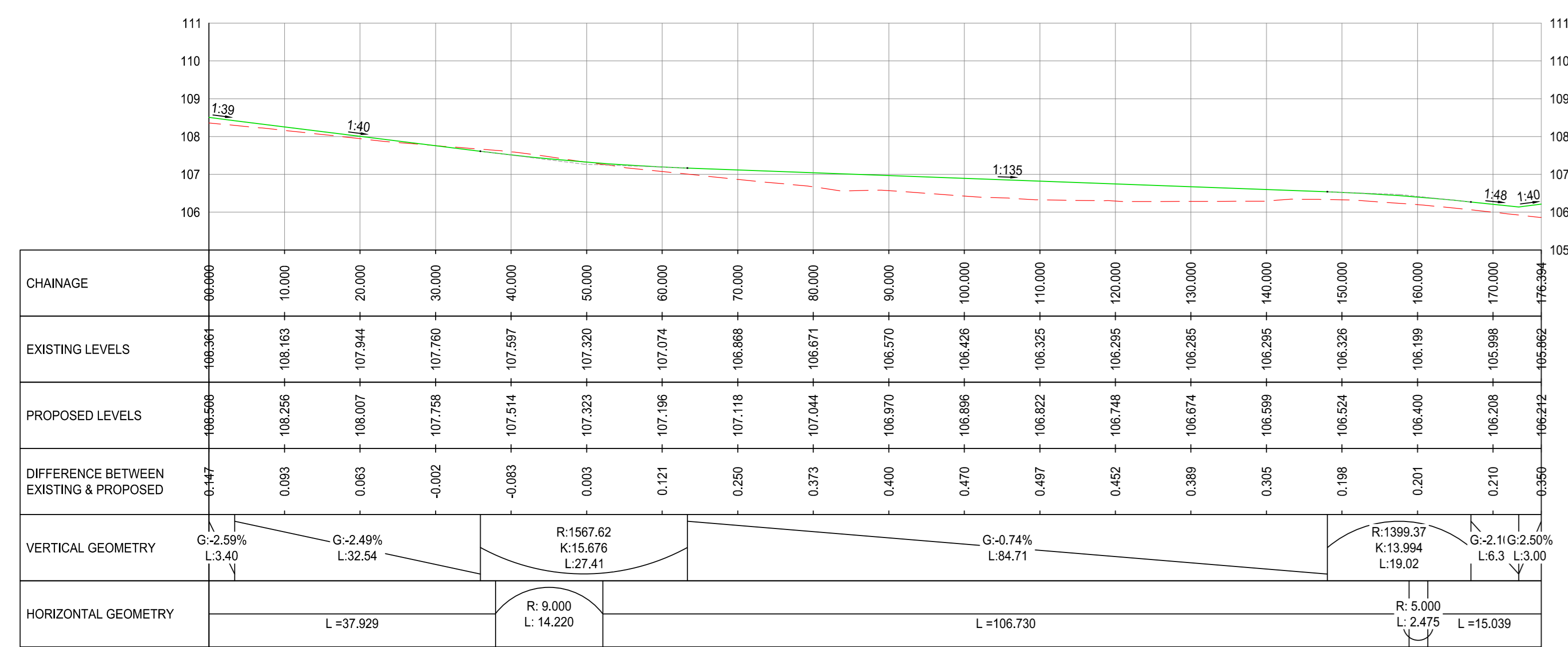
ALIGNMENT - (14) SCALE: H 1:500, V 1:100, DATUM: 105.000
